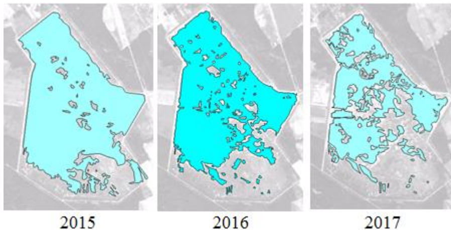
Сокращение площади водного зеркала Днепро-Брагинского водохранилища в 2014-2017 годах (по данным дистанционного зондирования, спутник Landsat-8, панхроматический канал)
